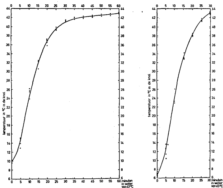
FIG. 20 Temperatuurverloop in 5 Bintje-knollen met kleinste diameter 40–45 mm, in water van 43° C en 45° C.
