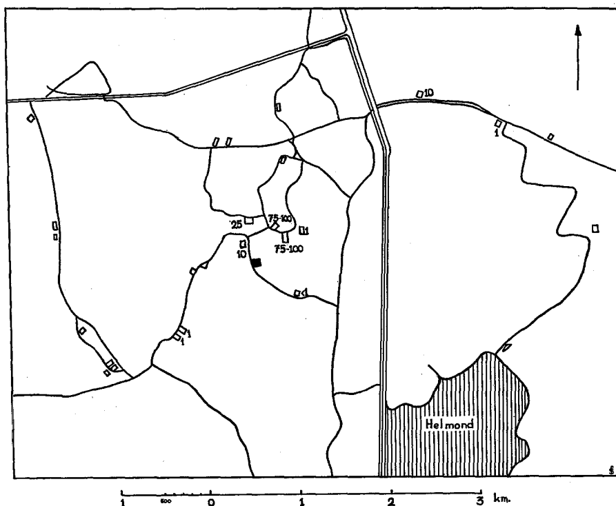
FIG. 15 Besmettingsgraad van percelen met Bintje in de omgeving van het veld met Wilpo (■) te Aarle-Rixtel op 21 juli 1954. Getallen geven percentage zieke blaadjes aan.
