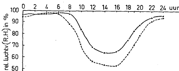
FIG. 17 2-uur gemiddelden van rel. luchtvochtigheid in en boven aard- appelgewas van 9-26 augustus 1955 (droge, winderige periode) 2-hour means of rel. humidity in and over potato crop from August 9-26, 1955 (dry windy period) — 10 cm boven de grond 10 cm above soil level - - - 2 m boven de grond 2 m above soil level
