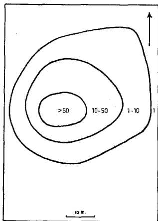
FIG. 14 Besmettingsgraad (% zieke planten) van een perceel met Wilpo te Aarle-Rixtel (N.B.) op 30 juni 1954
