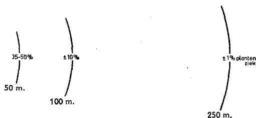
FIG. 13 Uitbreiding haard 2 in noord- oostelijke richting op 23 juni 1953
