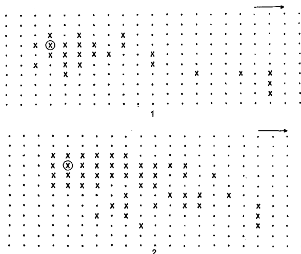
FIG. 12 Primaire haarden in percelen met Eersteling op 4 juni 1953 in De Streek
