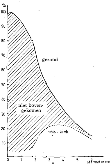
FIG. 11 Invloed afstand van inoculatieplek tot spruit op het percentage sec.-zieke planten (-----) en het percentage sec.-zieke planten + niet bovengekomen planten (—) Influence of distance from inoculation point to sprout, on the percentage of sec. diseased plants (-----), and the percentage of sec. diseased plants + plants not emerged (—)
