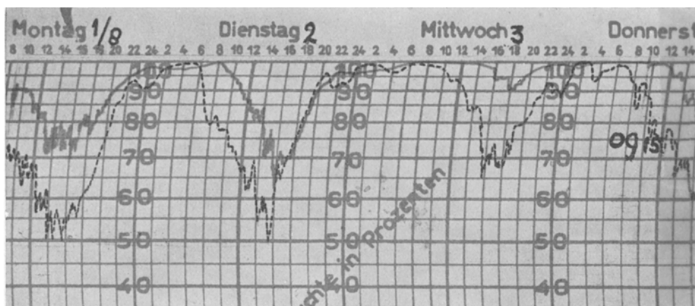
FIG 16. Strook van hygrograaf, geplaatst in aardappelgewas van 1-7 augustus 1955
